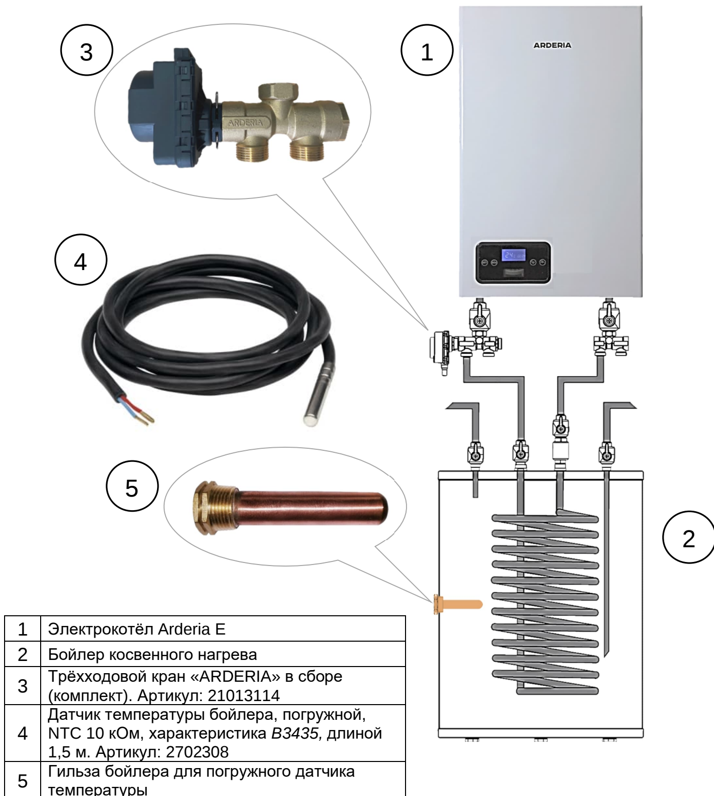
Рис. 25 схема подключения бойлера косвенного нагрева к электрокотлу.
