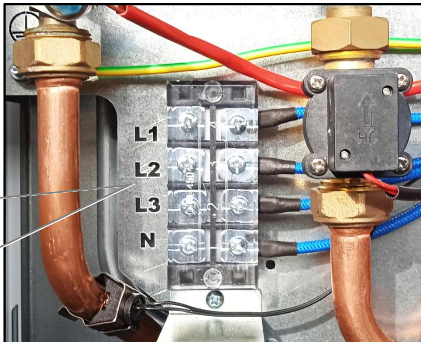
Рис. 14 Трёхфазное подключение
