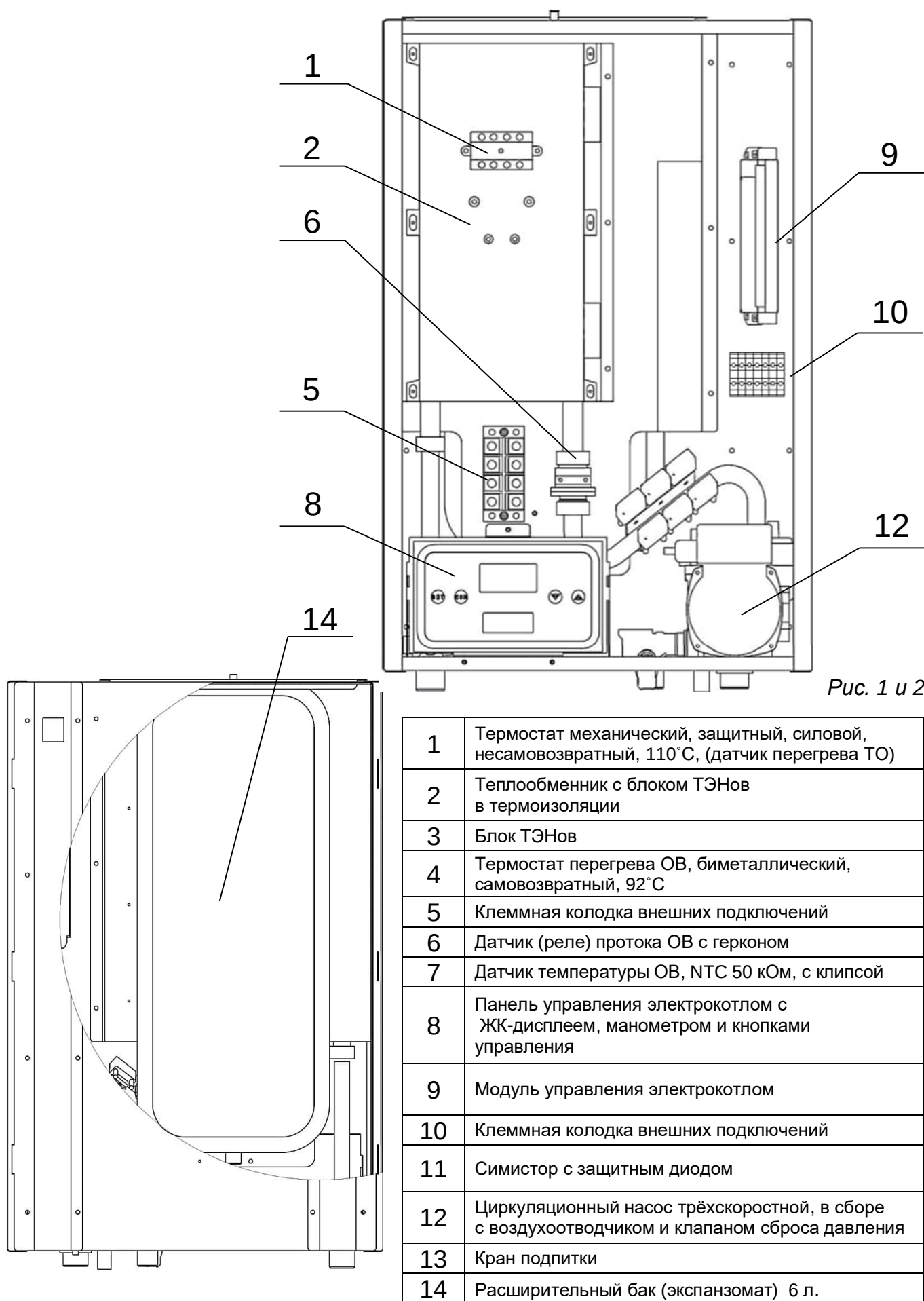
Рис. 2 Внутреннее устройство
