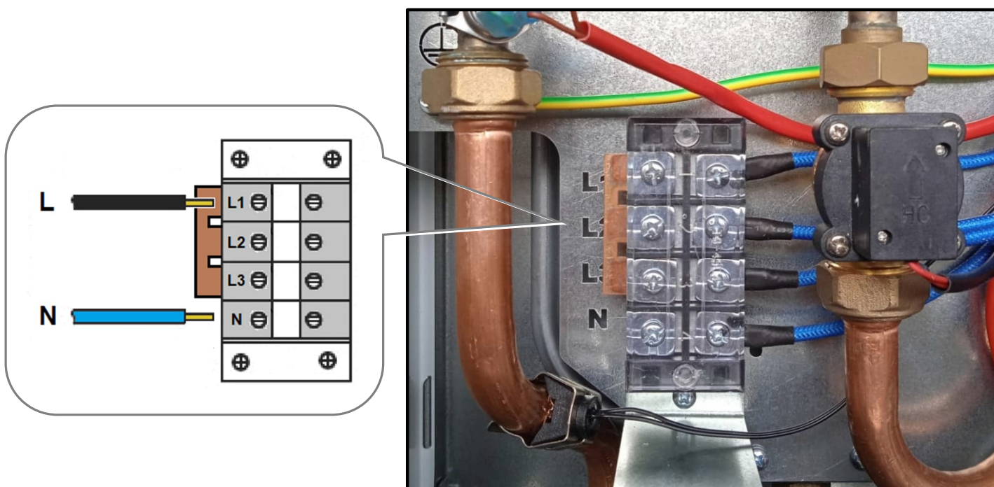
Рис. 15 Однофазное подключение
