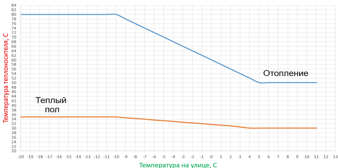
Рис 23. Графики компенсации уличной температуры.
