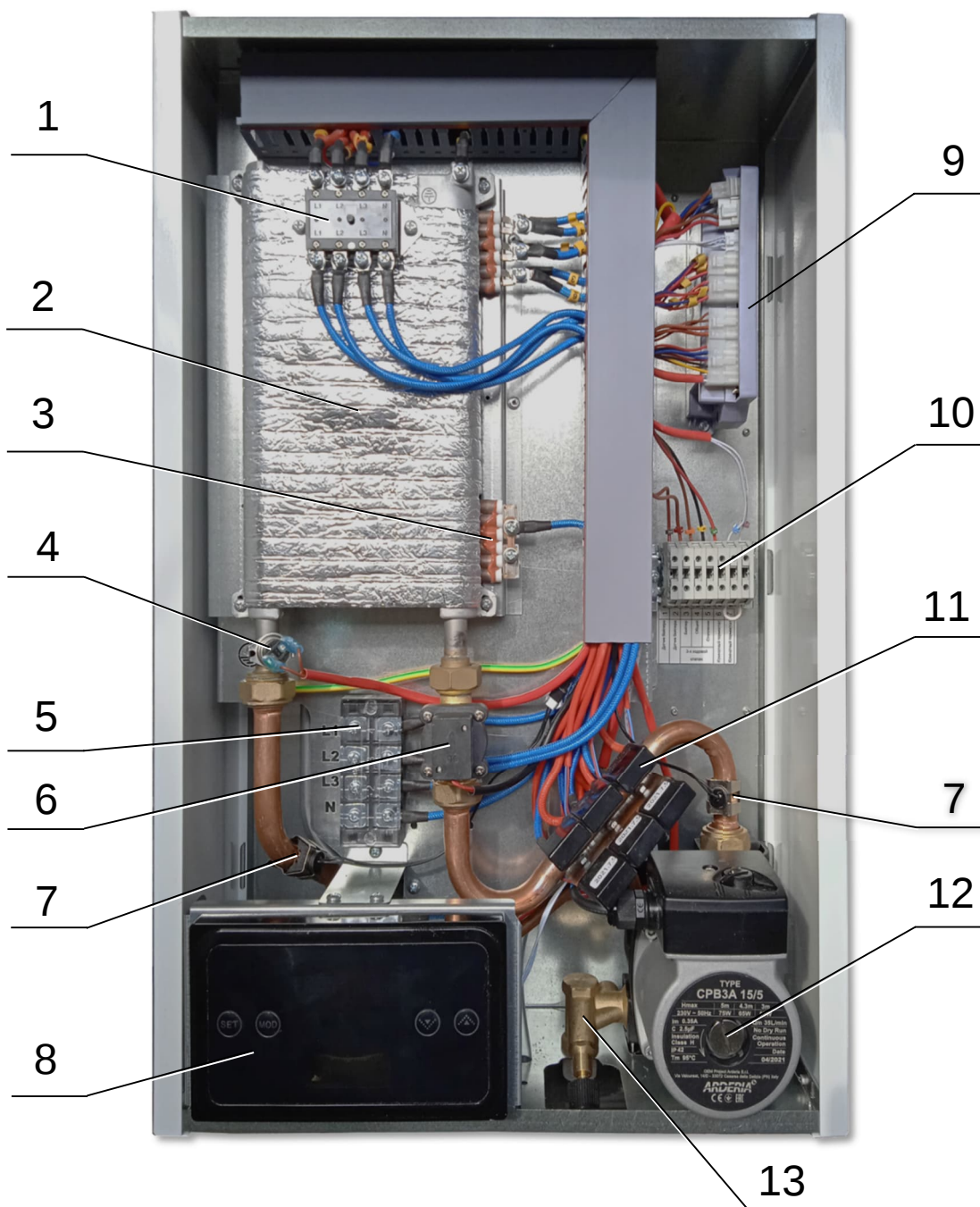
Рис. 1 Общий вид.
