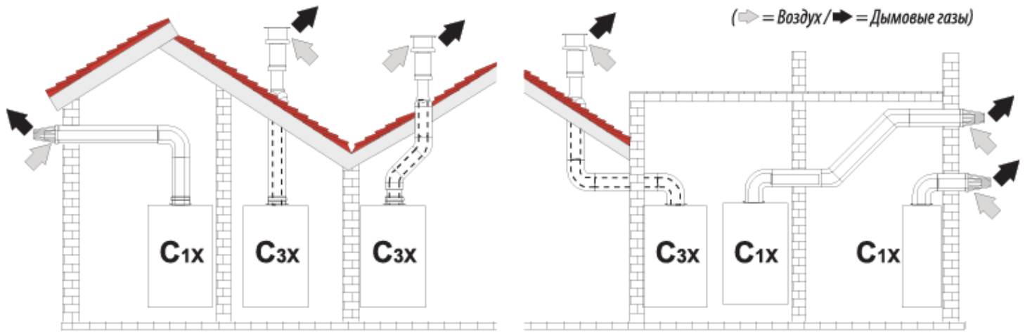
Примеры организации системы дымоудаления при помощи коаксиальных труб
