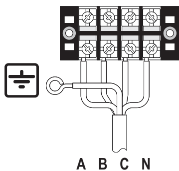
Рис. 3. Схема 3-фазного подключения электрокотла
